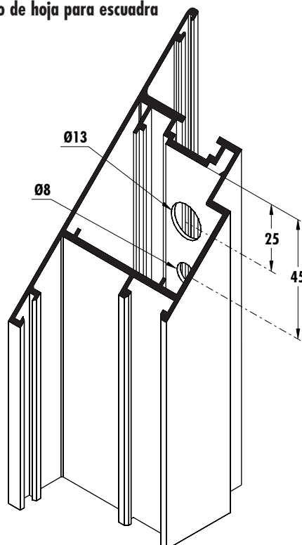
Mecanizado de hoja para escuadra
