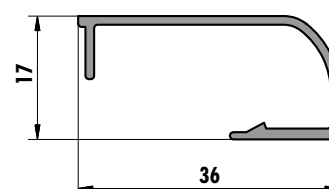
6257 (0,240 kg/m)
