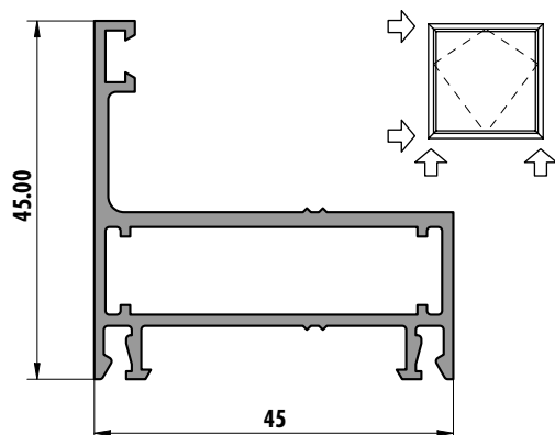
6259 (0,726 kg/m)
