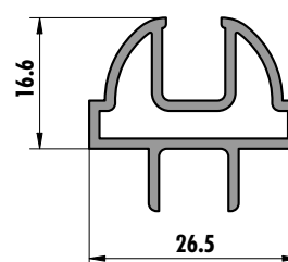
6267 (0,383 kg/m)
