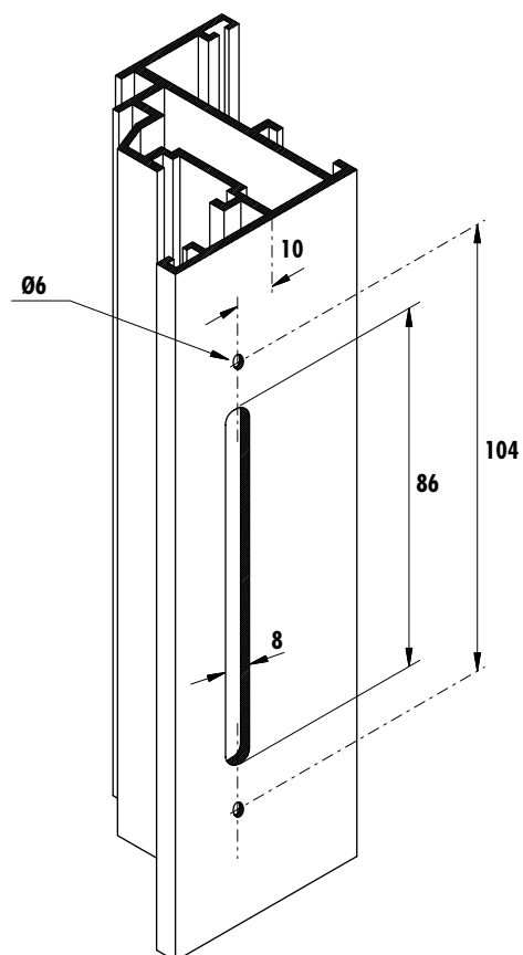
Mecanizado para H48
