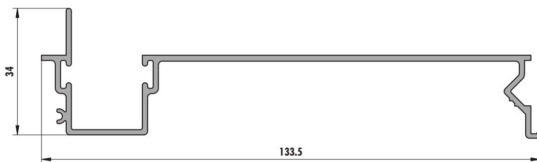
6244 (0,913 kg/m)
