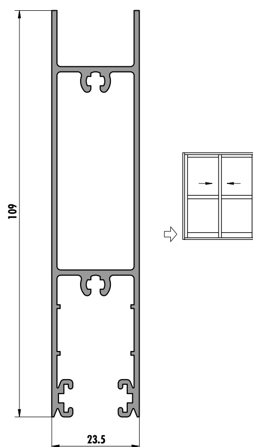
6252 (1,237 kg/m)
