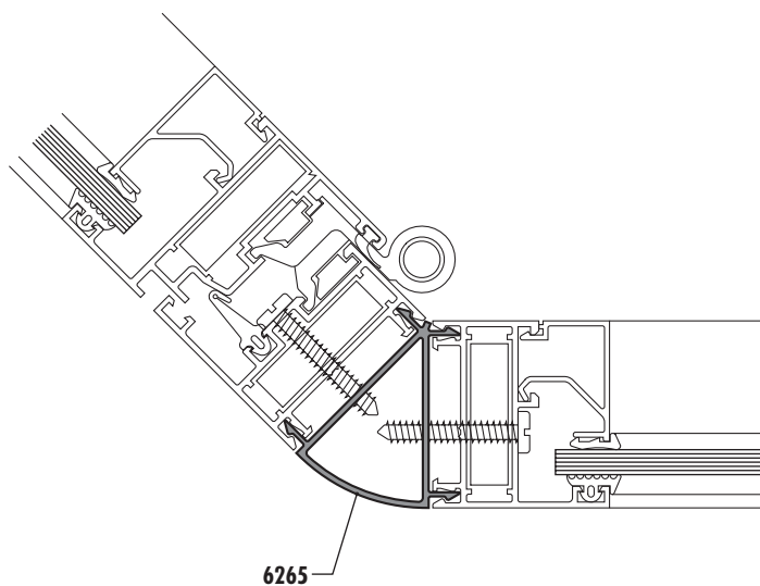
Perfil de acople a 135° Corte 1
