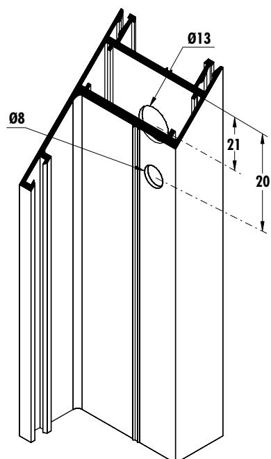
Mecanizado de marcos para escuadra
