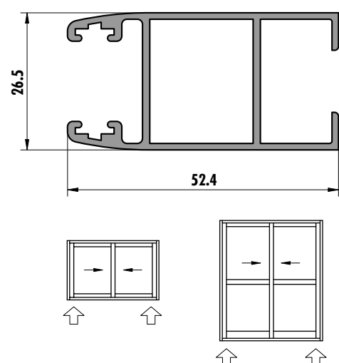
6203 (0,651 kg/m)
