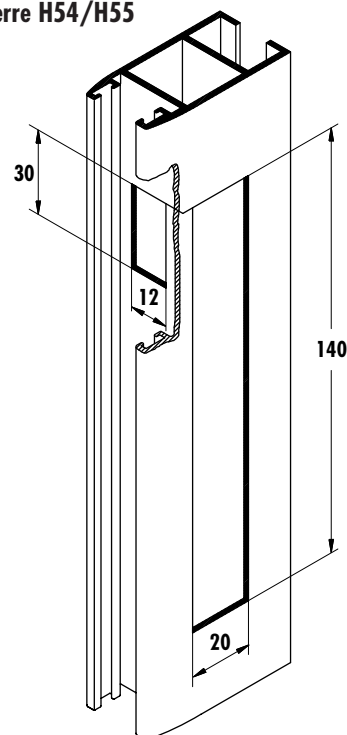
Mecanizado cierre H54/H55
