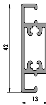
6256 (0,508 kg/m)
