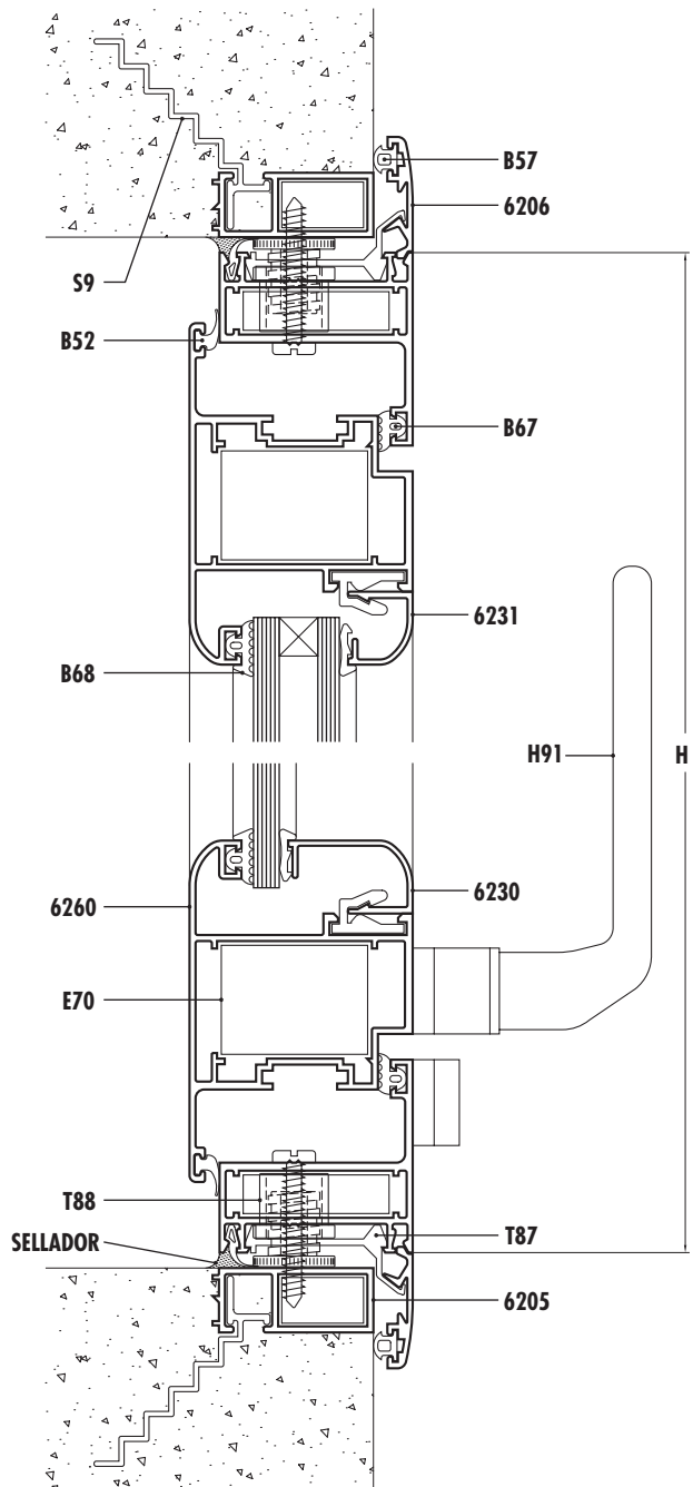
VPC Corte 5-6
