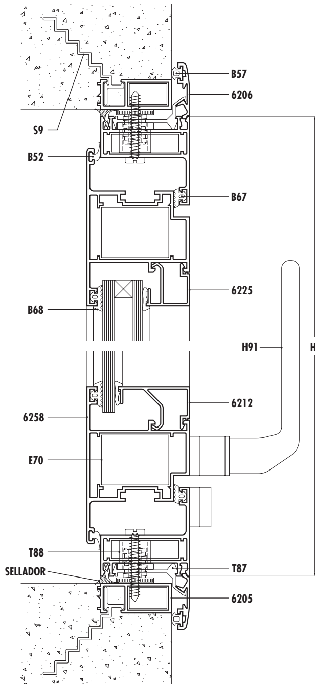
VPR Corte 1-2
