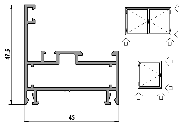
6210 (0,789 kg/m)
