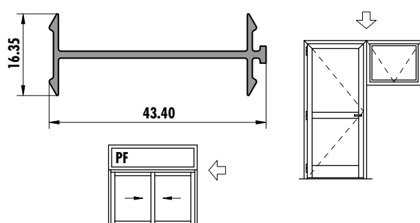
6213 (0,257 kg/m)
