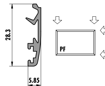
6206 (0,181 kg/m)
