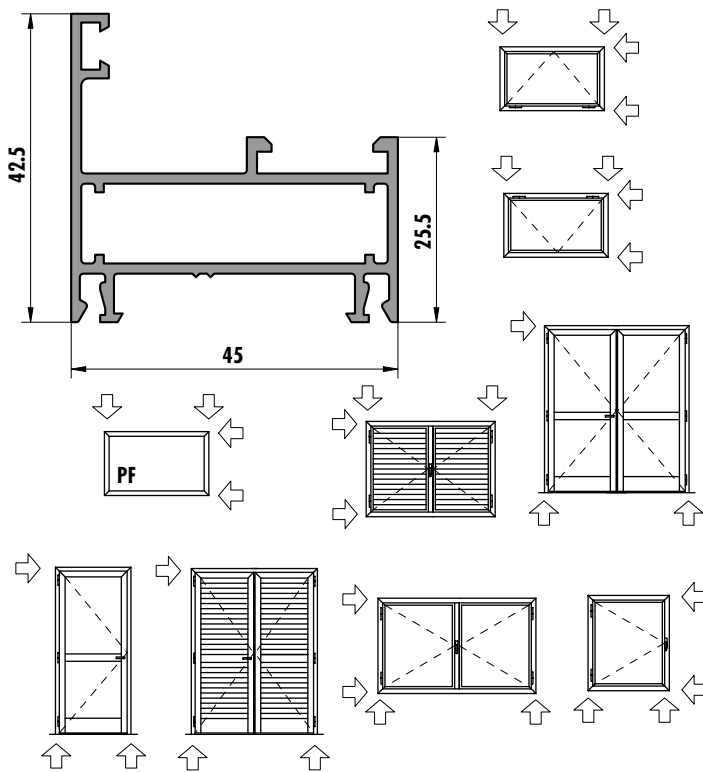
6216 (0,726 kg/m)
