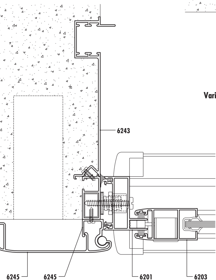
Detalle guía barro
