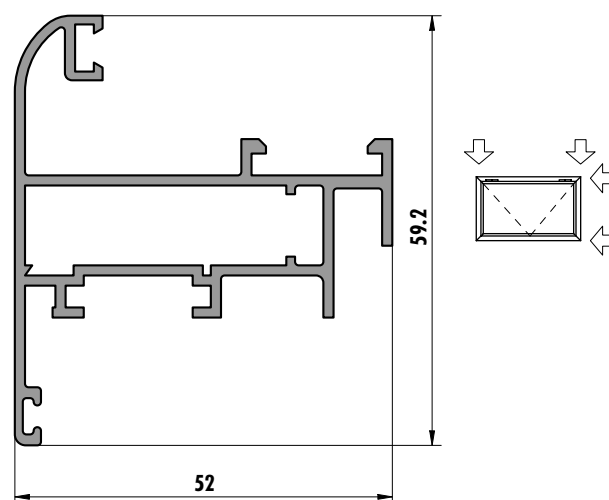
6236 (0,907 kg/m)
