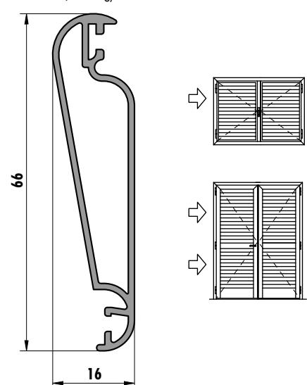
6277 (0,518 kg/m)
