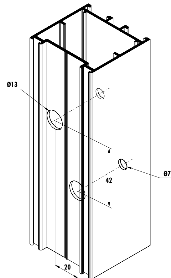
Mecanizado de marco para escuadra
