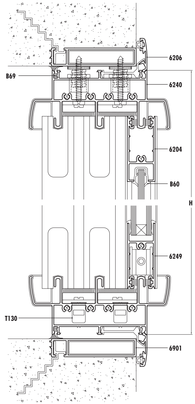
VPC3H Corte 9-10
