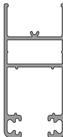
6909 (0,840 Kg/m)
