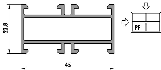
6270 (0,651 kg/m)
