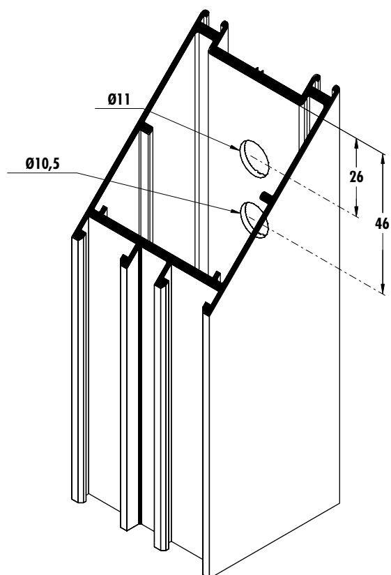
Mecanizado de hoja para escuadra
