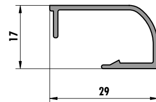
6230 (0,213 kg/m)
