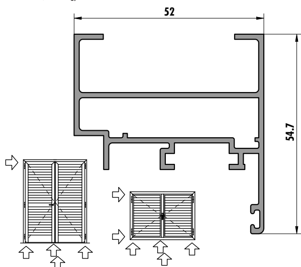
6275 (0,880 kg/m)
