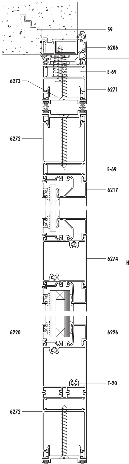
PVVR Corte 1-2-3
