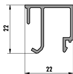
6225 (0,257 kg/m)
