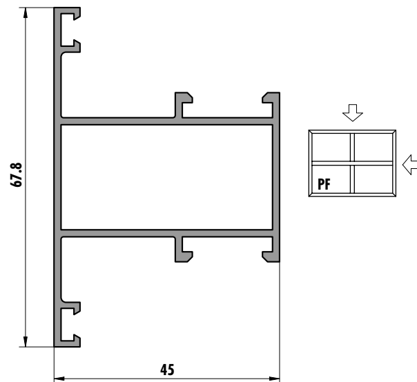
6222 (0,842 kg/m)
