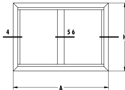
PFR paño fijo recto
