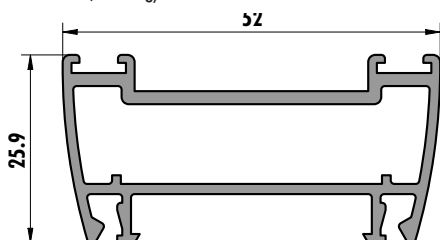
6286 (0,740 kg/m)
