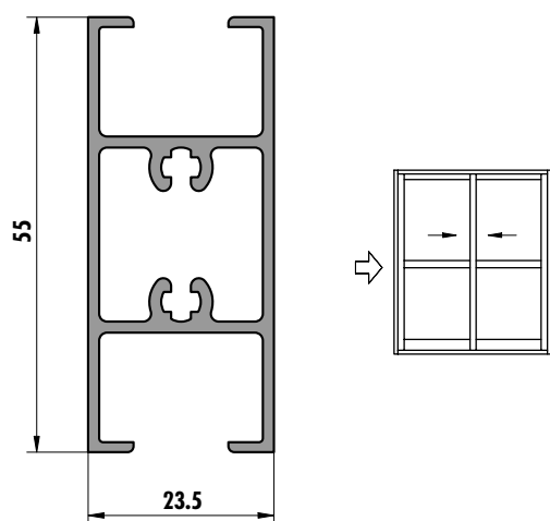
6239 (0,705 kg/m)
