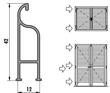
6278 (0,319 kg/m)
