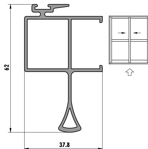
6251 (0,797 kg/m)
