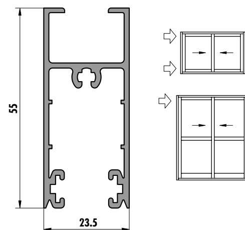
6204 (0,705 kg/m)
