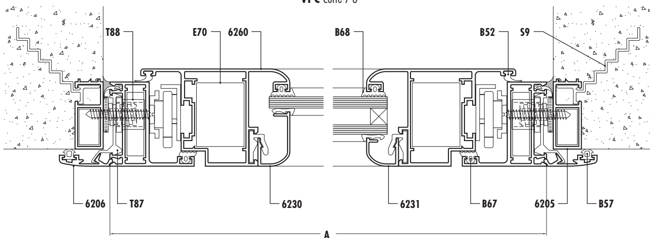
VPC Corte 7-8
