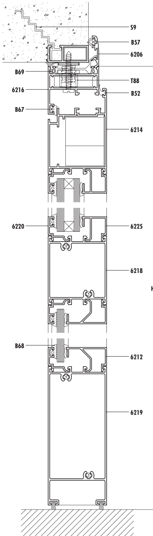
PRR Corte 1-2-3
