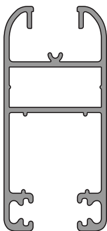
6908 (0,894 Kg/m)
