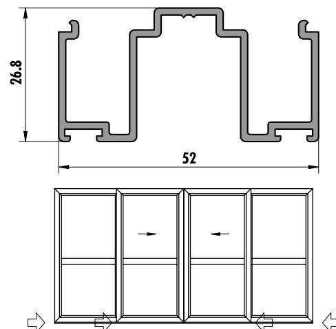
6282 (0,605 kg/m)
