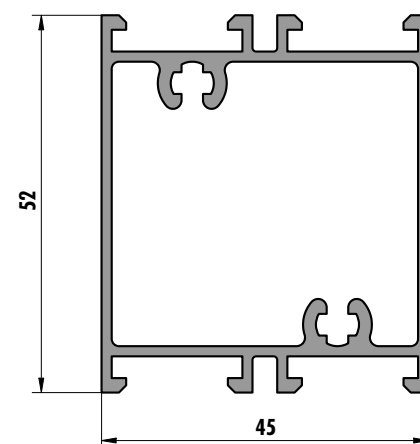
6274 (1,039 kg/m)
