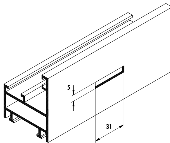
Mecanizado para drenaje
