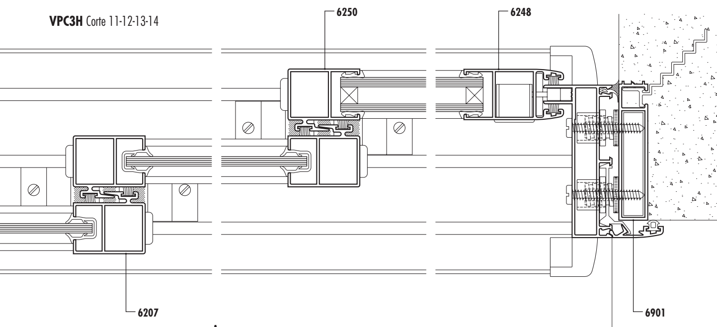
VPCVR Corte 15-16
