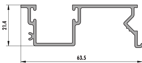
6243 (0,548 kg/m)
