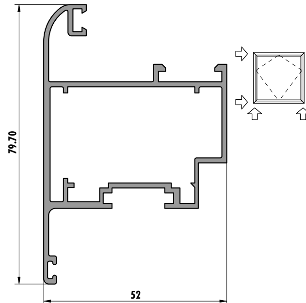
6260 (1,099 kg/m)
