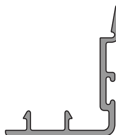
6907 (0,338 Kg/m)
