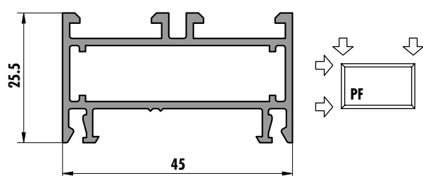
6269 (0,670 kg/m)
