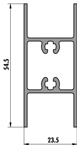
6253 (0,689 kg/m)
