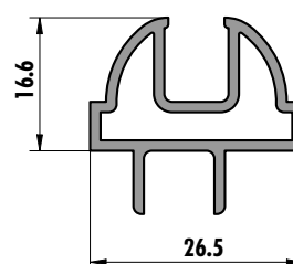
6266 (0,383 kg/m)
