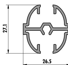
6268 (0,429 kg/m)
