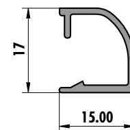
6231 (0,170 kg/m)
