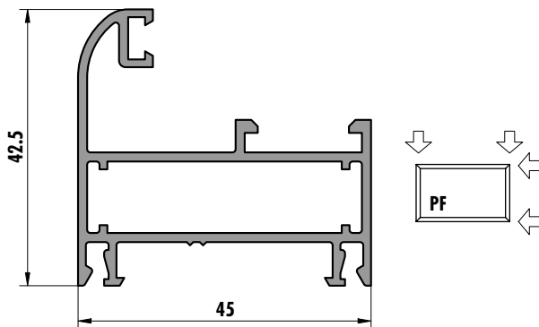
6229 (0,764 kg/m)
