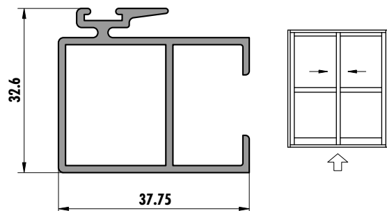
6207 (0,613 kg/m)
