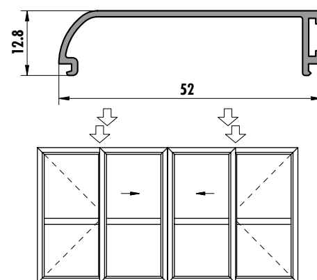
9284 (0,257 kg/m)
