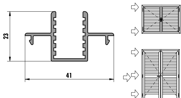
6280 (0,367 kg/m)
