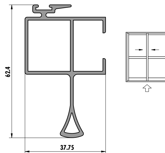
6208 (0,813 kg/m)
