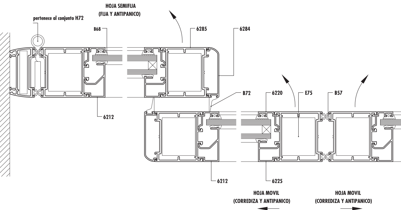
PCAAR Corte 4-5-6
