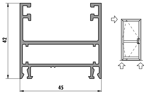
6271 (0,880 kg/m)
