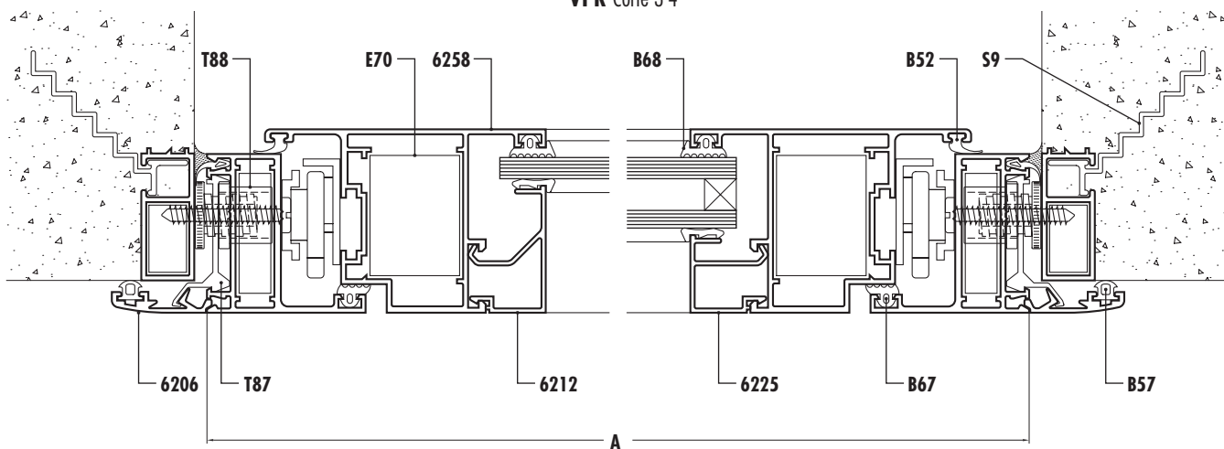
VPR Corte 3-4
