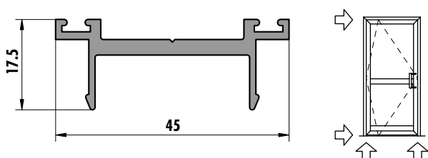
6273 (0,456 kg/m)
