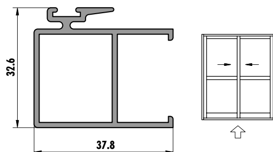
6250 (0,583 kg/m)
