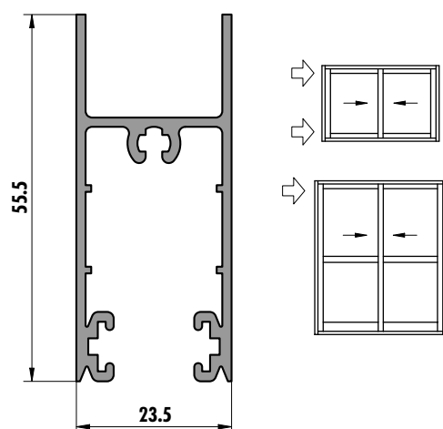
6249 (0,689 kg/m)
