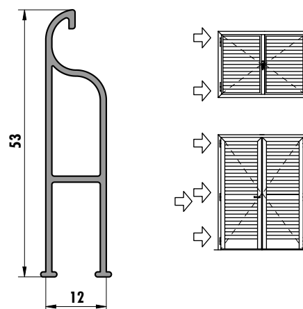
6279 (0,392 kg/m)
