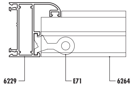
Detalle ensamble con travesaño
