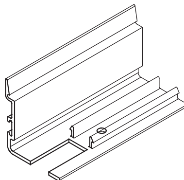
Mecanizado suplemento parante central
