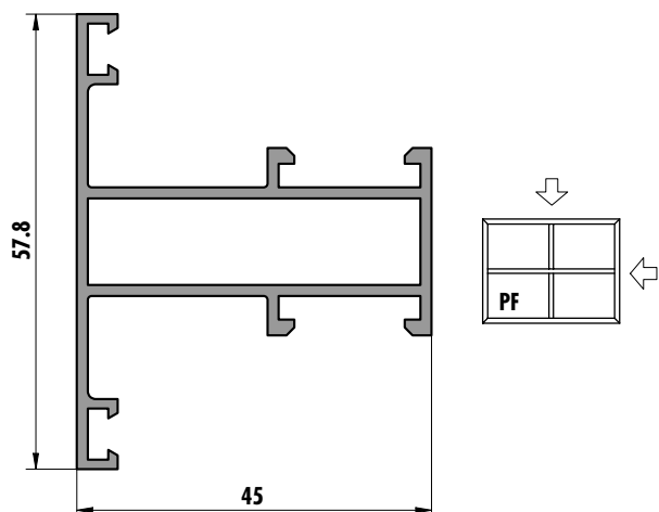
6221 (0,767 kg/m)
