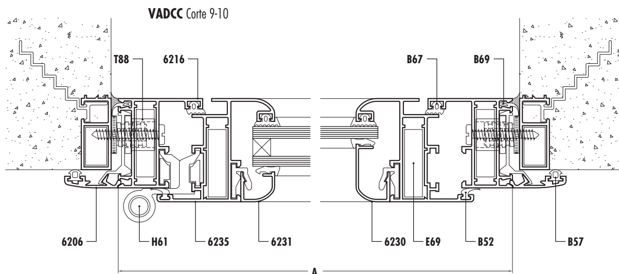
VADCR2 Corte 11-12-13
