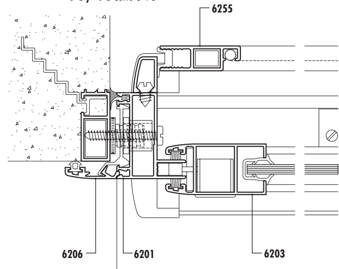
VPC3H Corte 9-10
