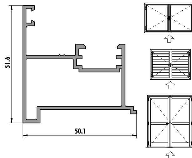
6224 (0,794 kg/m)
