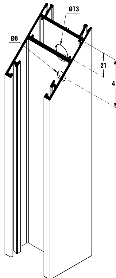
Mecanizados escuadra hoja
