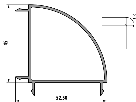
6262 (0,680 kg/m)
