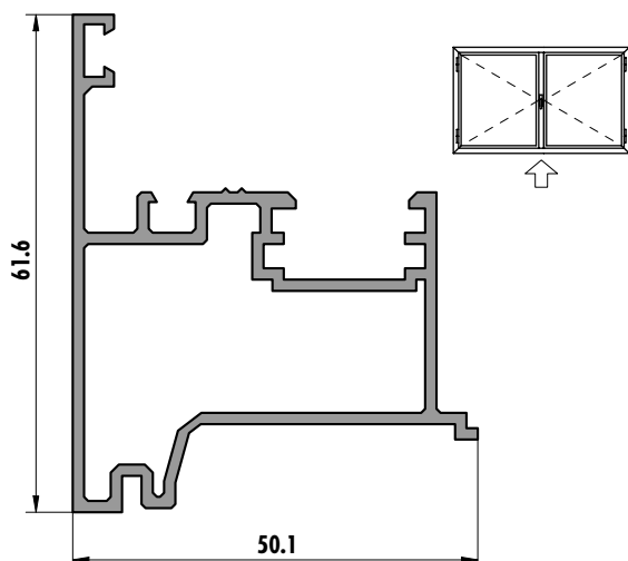
6223 (0,918 kg/m)
