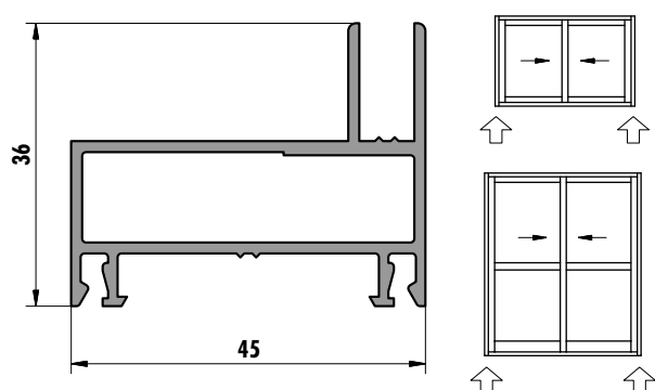
6201 (0,664 kg/m)
