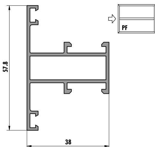
6264 (0,713 kg/m)
