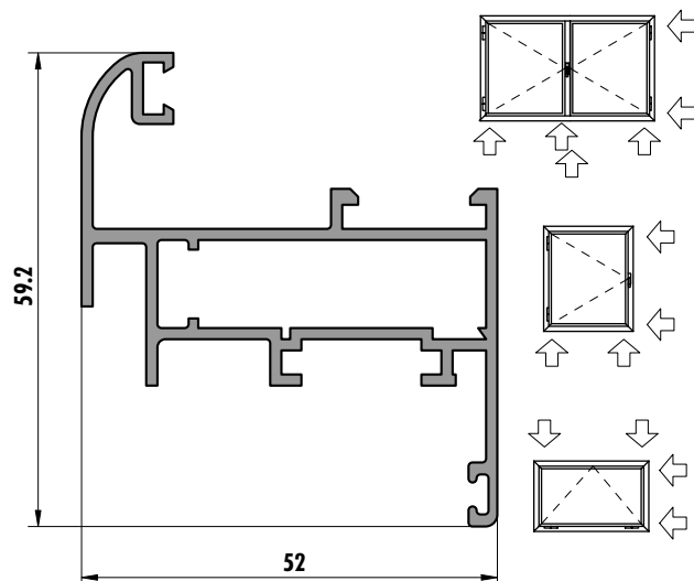
6235 (0,902 kg/m)
