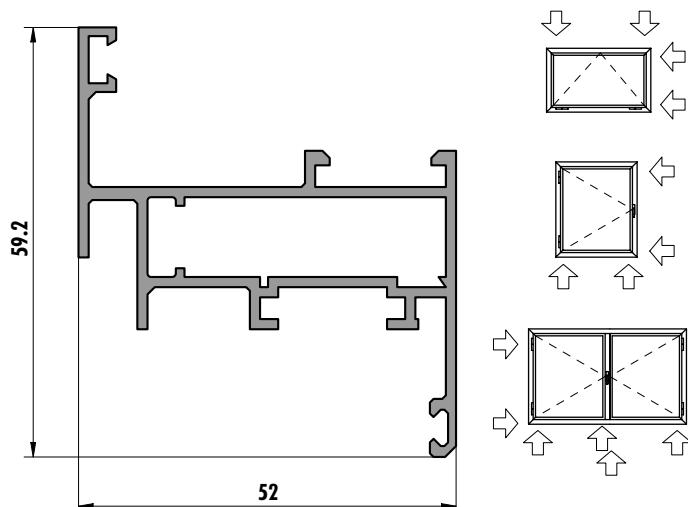
6215 (0,864 kg/m)
