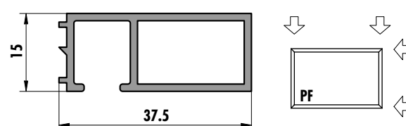
6205 (0,410 kg/m)
