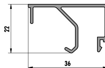
6212 (0,316 kg/m)
