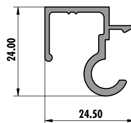
6254 (0,302 kg/m)
