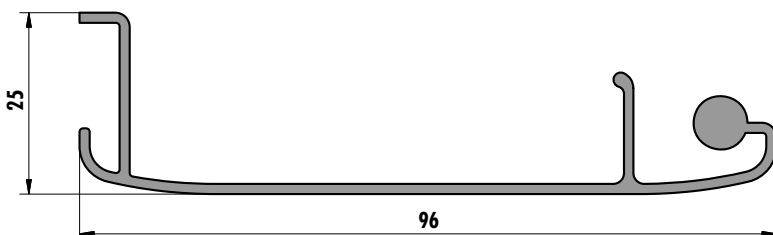
6245 (0,678 kg/m)
