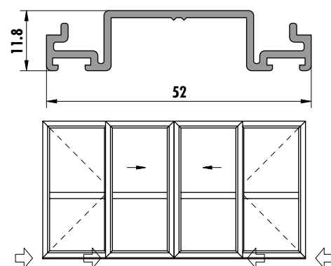
6283 (0,381 kg/m)
