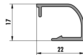
6232 (0,194 kg/m)
