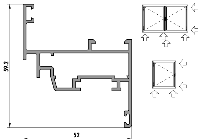
6211 (0,848 kg/m)
