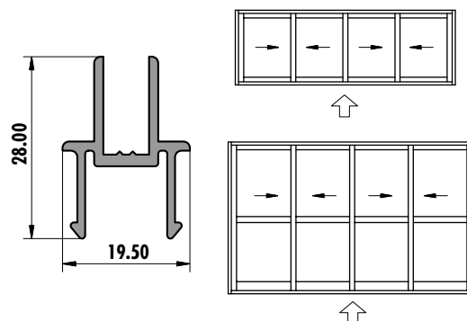
6246 (0,292 kg/m)
