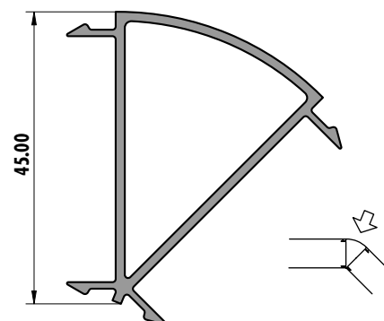
6265 (0,543 kg/m)
